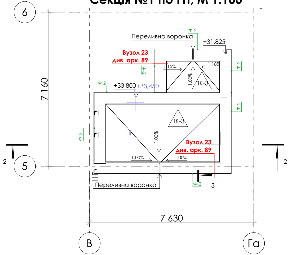
План покрівлі над сходовою. Секція №1 по ГП, М 1:100
