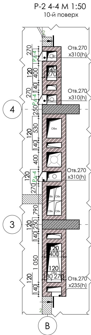
Розгортка вентканалу P-2 М 1:50
