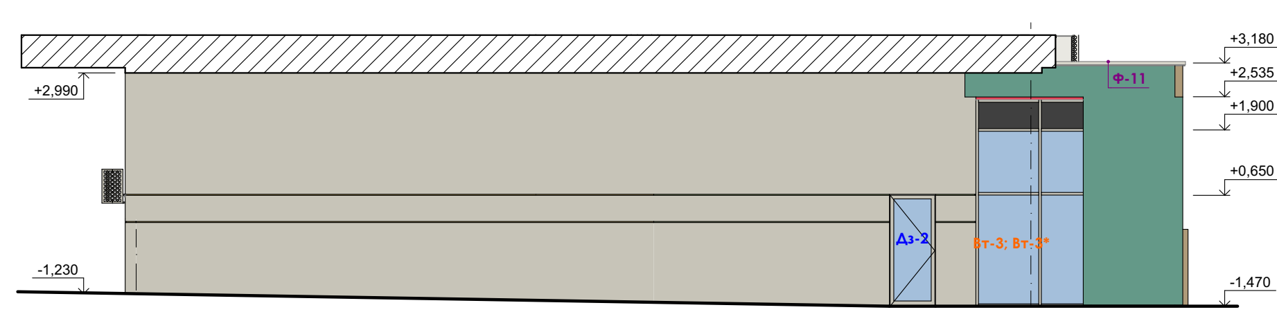
Фасад в осях Аа-Га. М 1:100
