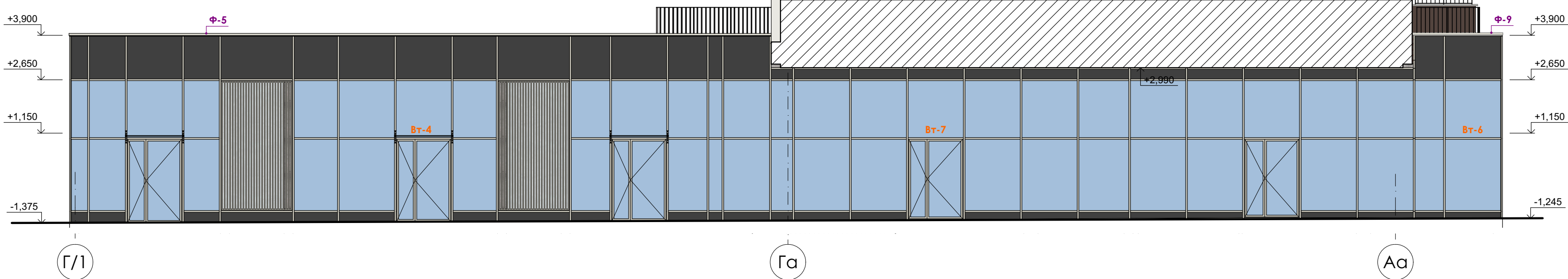
Фасад в осях Г/1-Аа. М 1:100
