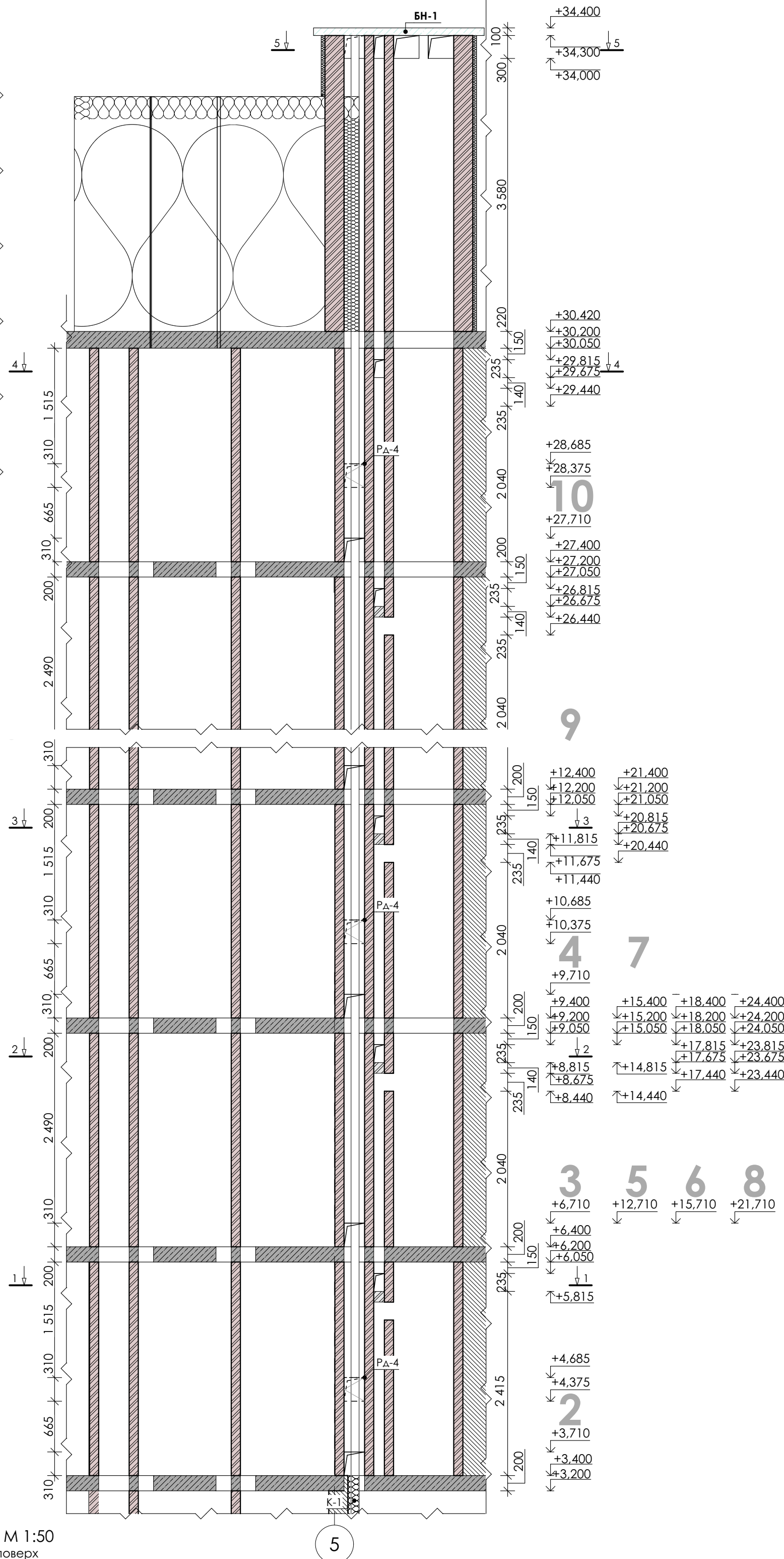
Розгортка вентканалу P-1 М 1:50
