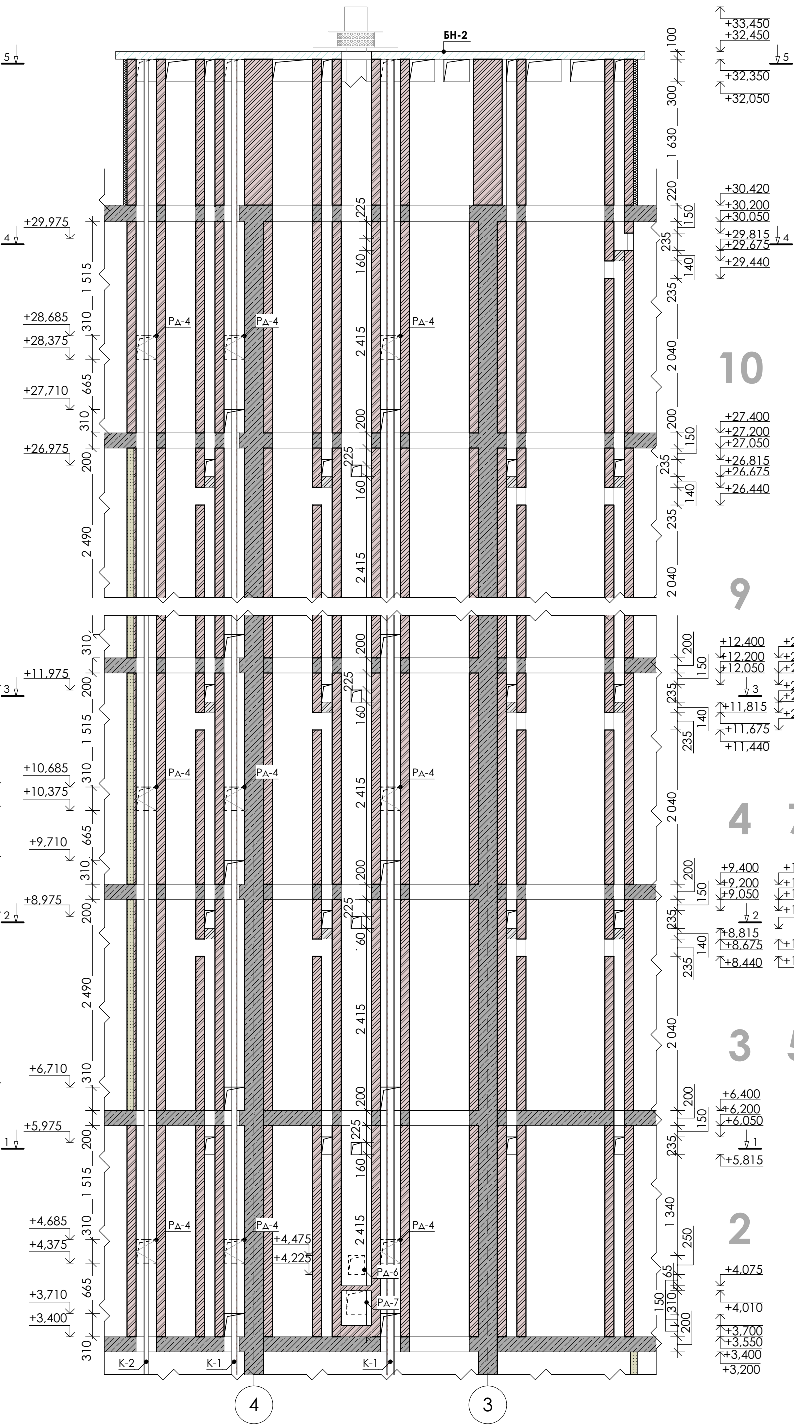
Розгортка вентканалу P-2 М 1:50
